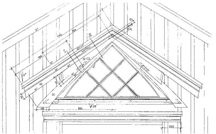
Detalj, gavelfönster.
