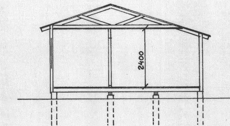
SEKTION
