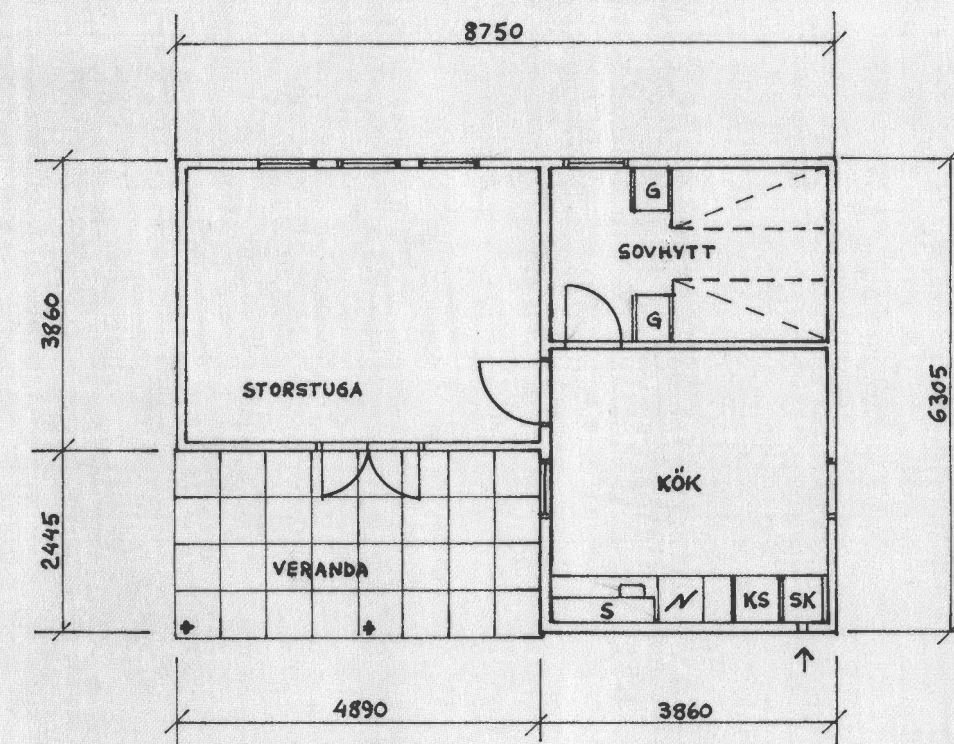
BOTTENPLAN YTA 43,4 M 2
