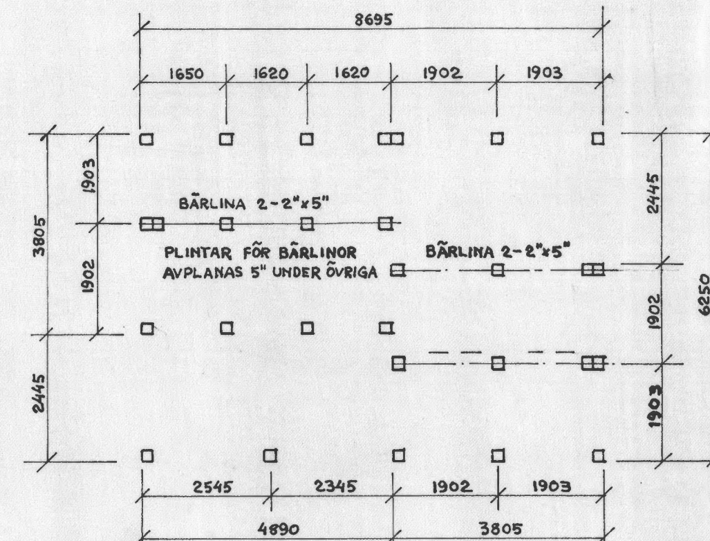
GRUNDPLAN
