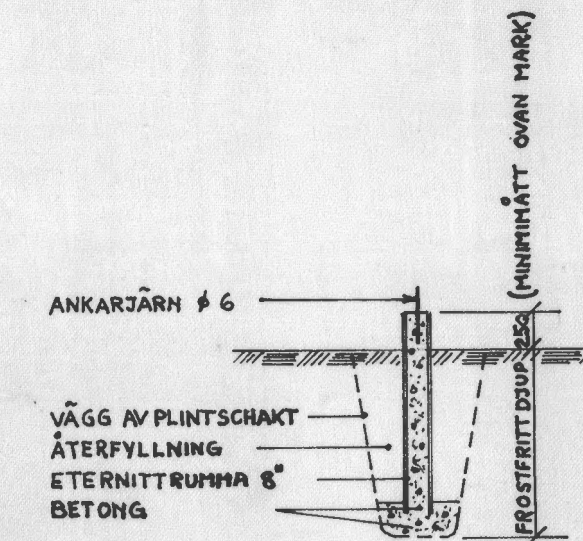
PRINCIPDETALJ AV GRUNDPLINT
