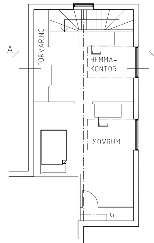
PLAN OVANVÅNING
