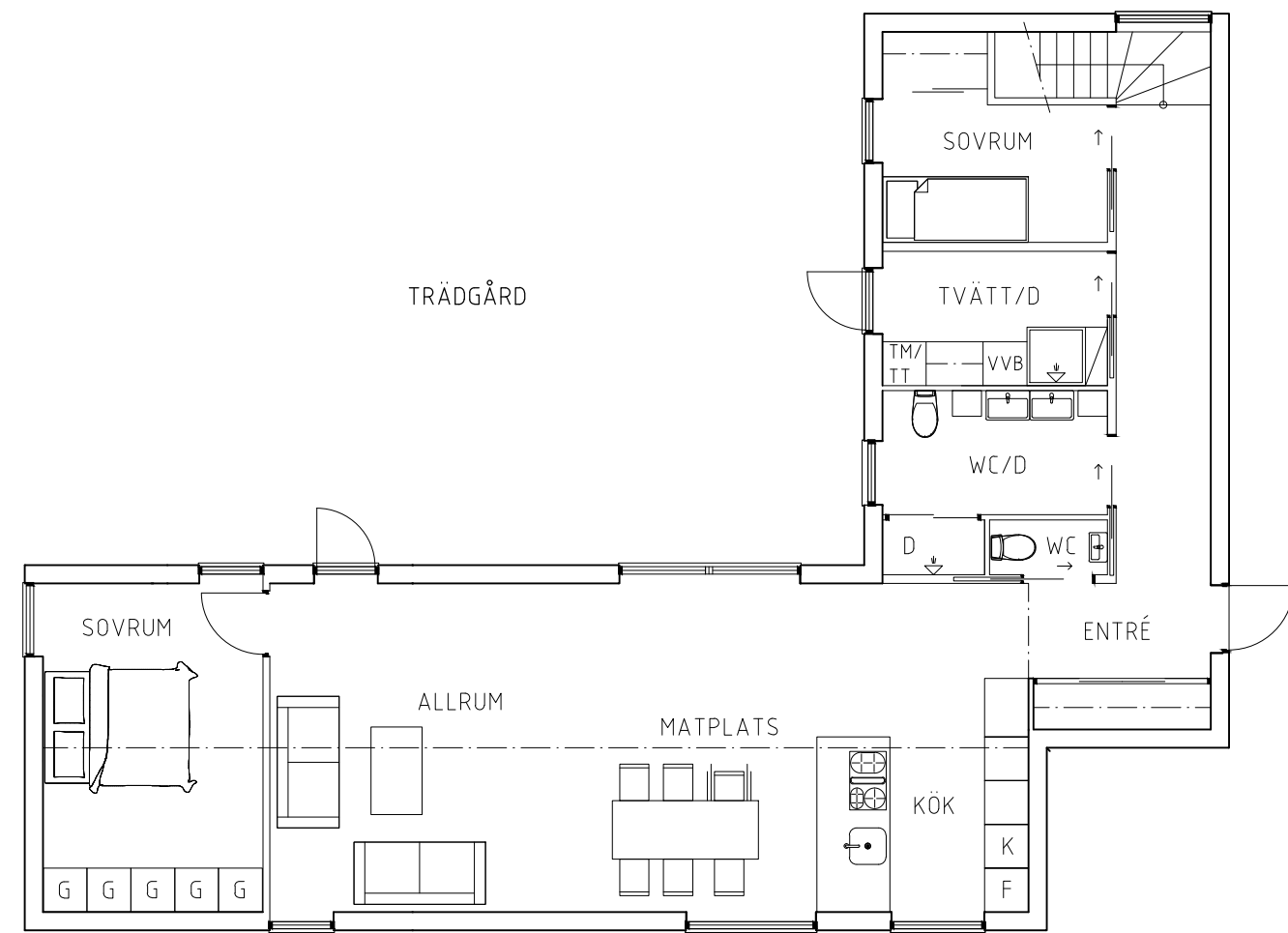
PLAN BOTTENVÅNING
