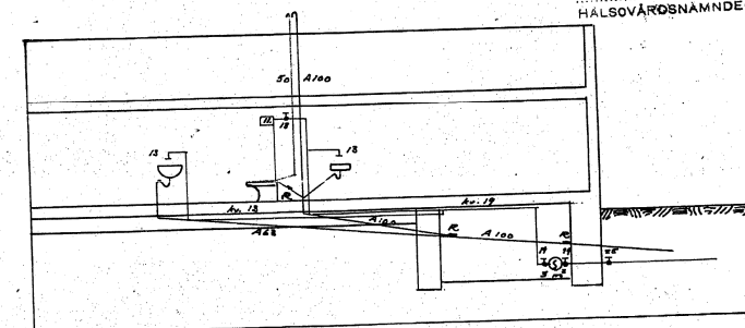
Schematisk sektion.
