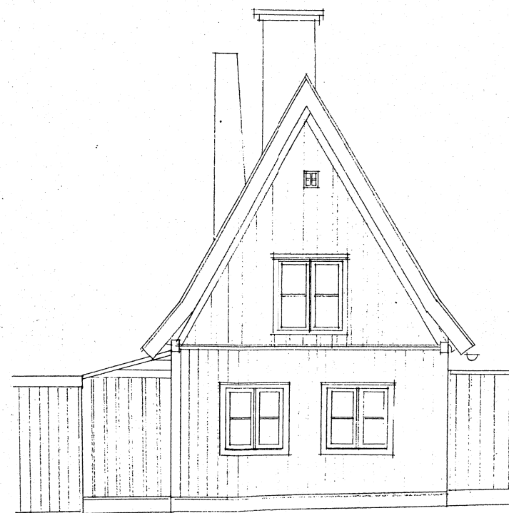
FASAD MOT MELLANGATAN, NORDVÄST - 1:50 -
