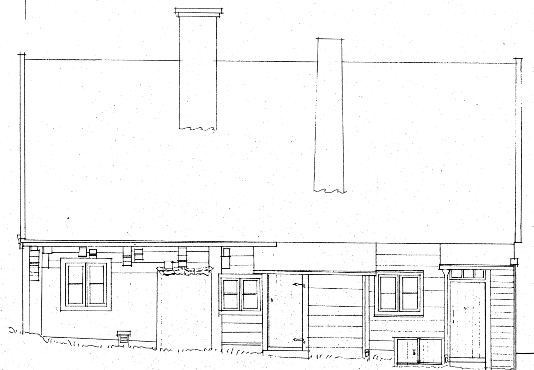
FASAD MOT GÅRDEN, NORDÖST - 1:50 -
