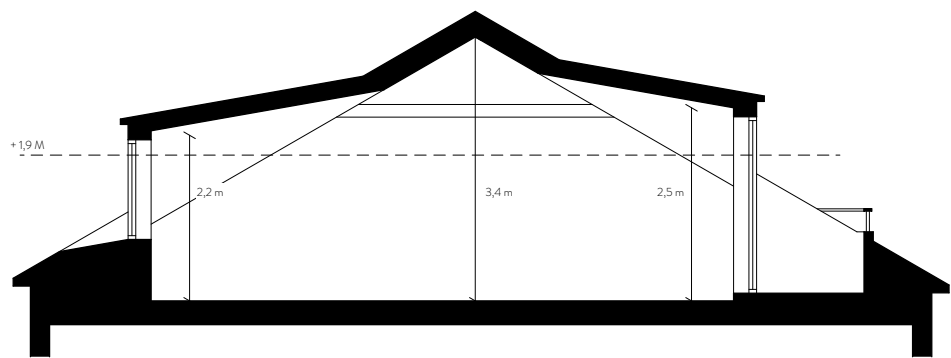
TVÄRSEKTION GENOM LÄGENHETEN
